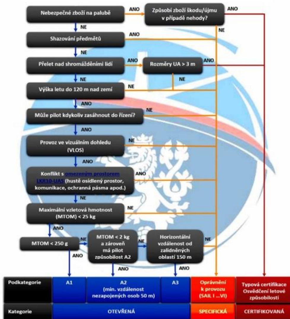
Obr. č. 2: Kategorizace provozu bezpilotních systémů
